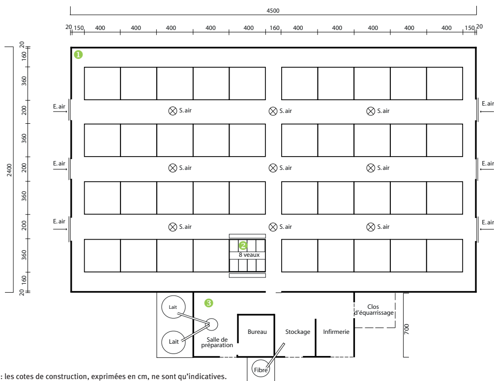
Plan I.1 : Plan de masse du bâtiment dur de 320 places
