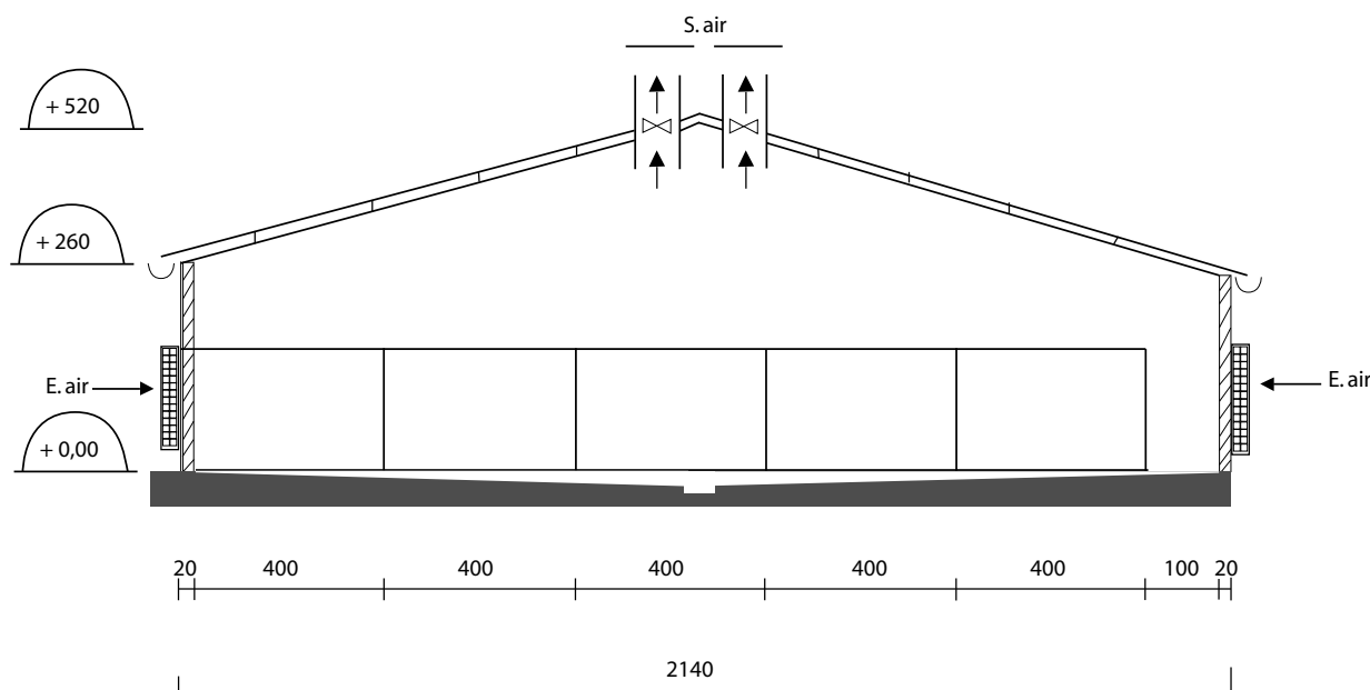
Plan III.2 : Vue en coupe du bâtiment dur de 300 places
