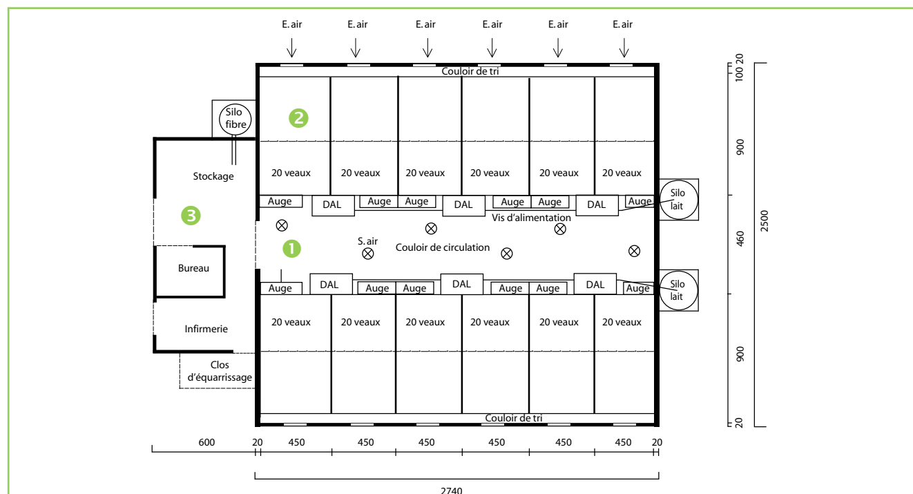
Plan IV.1 : Plan de masse du bâtiment dur de 240 places
