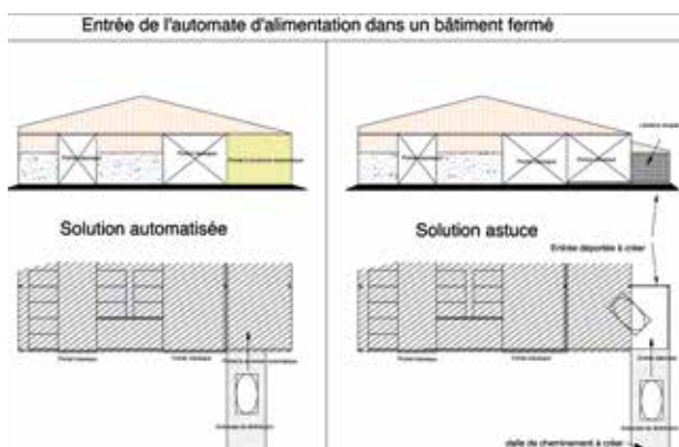
Schéma 11.1 : Principe de l'accès déporté
