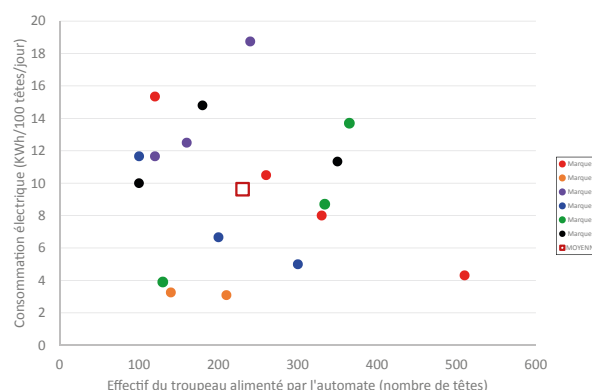
Graphique 10.1 : Consommation électrique annoncée par les marques selon l'effectif du troupeau alimenté par le robot d'alimentation
