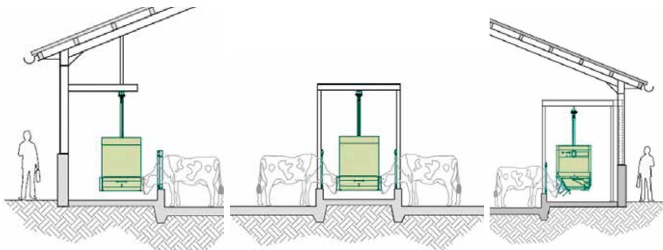
Figure 7.1 : Exemples d'adaptation du rail à la charpente (existant/neuf) – Source GEA
