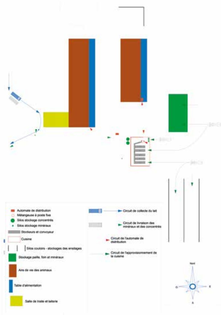
Plan 6.1 : Exemple de cuisine indépendante du logement des animaux avec un automate de distribution sur roues
