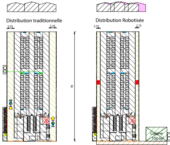
Plan 11.2 : Plans de principe d'une stabulation de 150 vaches laitières avec deux couloirs d'alimentation latéraux pour une distribution traditionnelle de l'alimentation et une distribution robotisée - Projet 2
