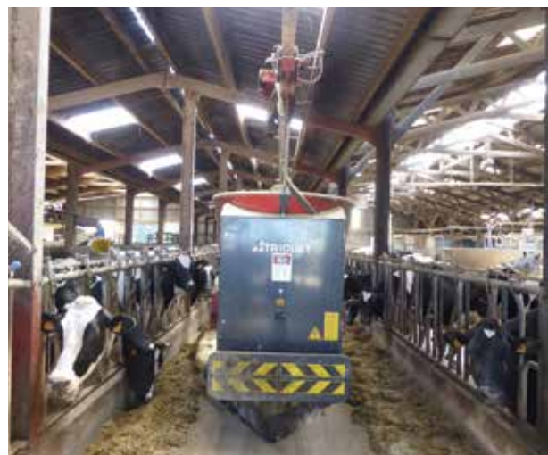
Photo 7.6 : Un couloir d'alimentation réduit ici à 3,10 m de large avec un rail central unique pour un fonctionnement de l'automate en va-et-vient avec distribution des deux côtés
