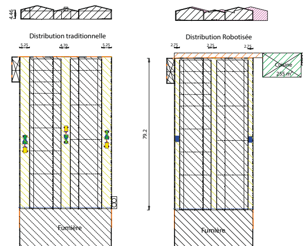
Plan 11.1 : Plans de principe d'une stabulation de 250 mètres/veaux avec distribution traditionnelle et distribution robotisée – Projet 1
