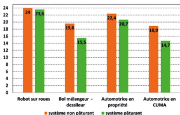
Graphique 11.9 : Comparaison des coûts totaux annuels pour un troupeau nourri de 300 têtes entre 4 modes de distribution de l'alimentation et pour deux systèmes, pâturant et non pâturant
