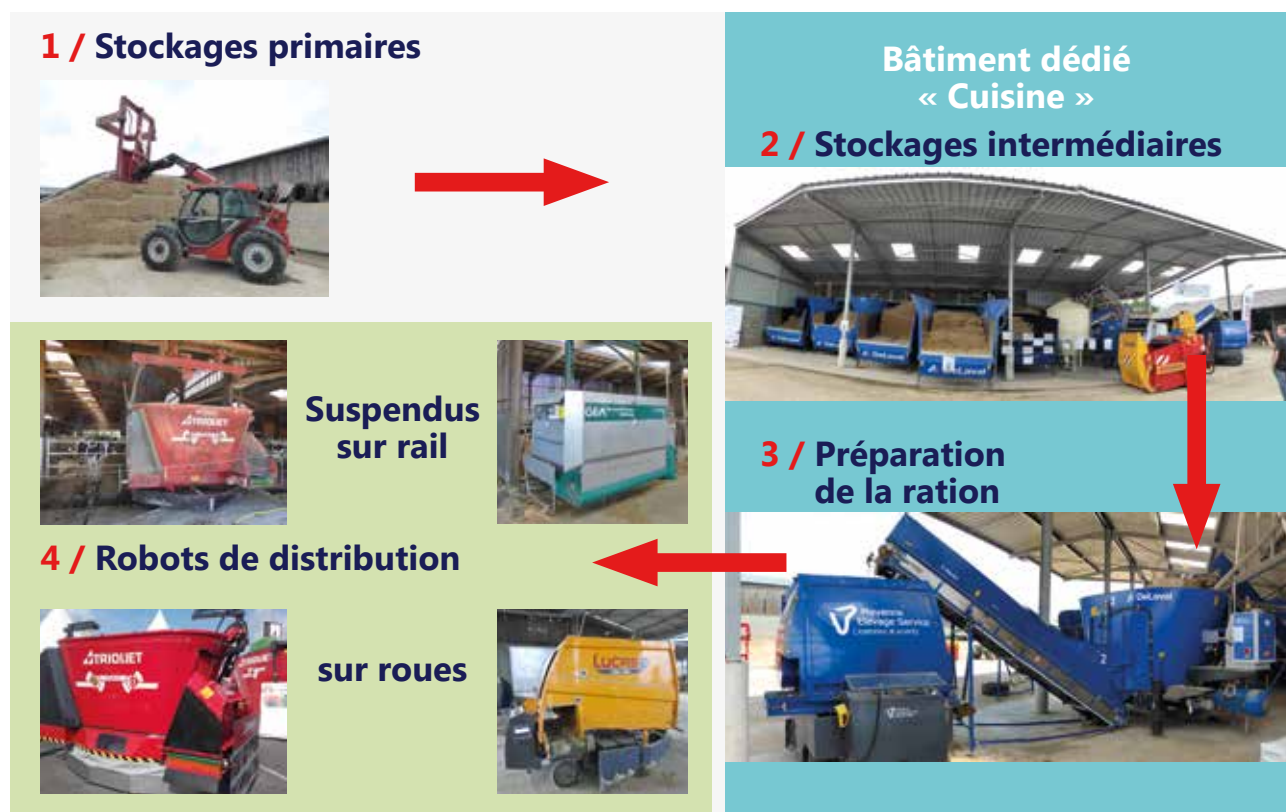
Figure 5.1 : Schéma de principe du mode de fonctionnement de l'automatisation de l'alimentation
