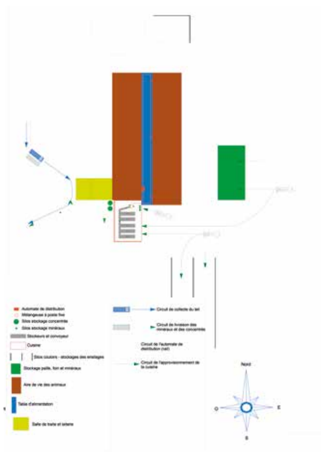
Plan 6.2 : Exemple de cuisine jouxtant en pignon le logement des animaux avec un automate de distribution sur rail
