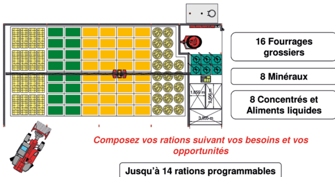
Plan 6.6 : Exemple d'aménagement interne d'une cuisine DeLaval (Famille D) - Source Lely.
