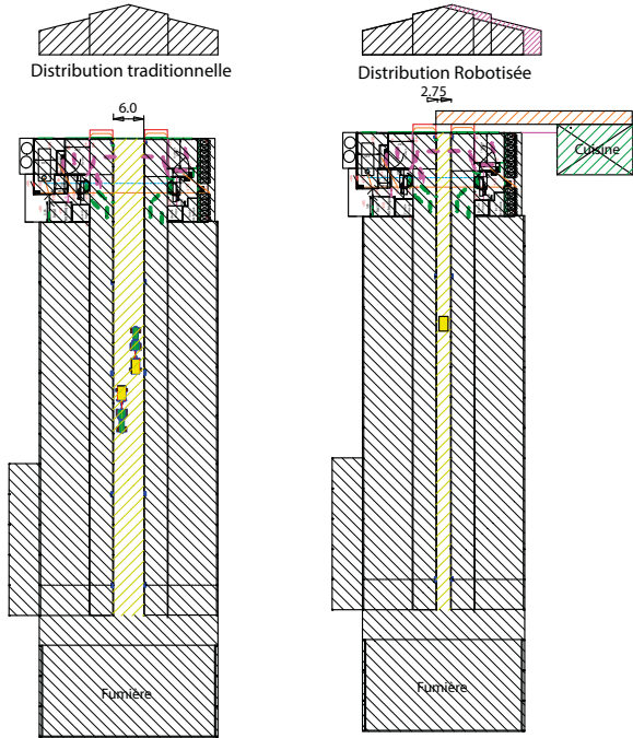
Plan 11.3 : Plans de principe d'une stabulation de 150 vaches laitières avec couloir d'alimentation central pour une distribution traditionnelle de l'alimentation (à gauche) et une distribution robotisée (à droite) - Projet 3
