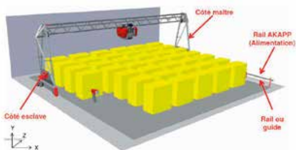
Photo 6.2 : Représentation 3D d'une cuisine équipée d'un portique mobile - Source Lely.
